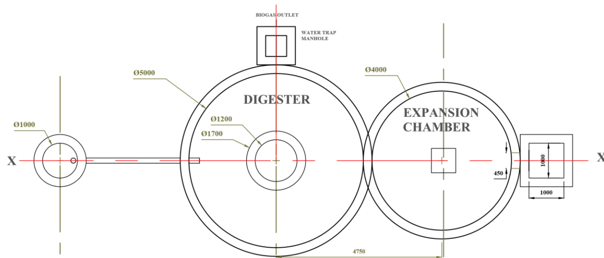
LAYOUT PLAN SCALE 1 : 50
